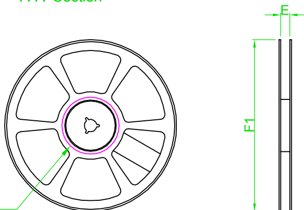
A-A' Section
