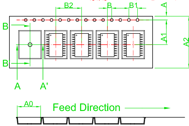
A-A' Section
