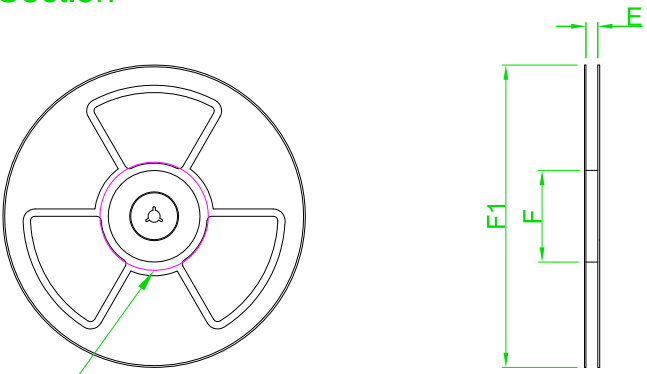
A-A' Section
